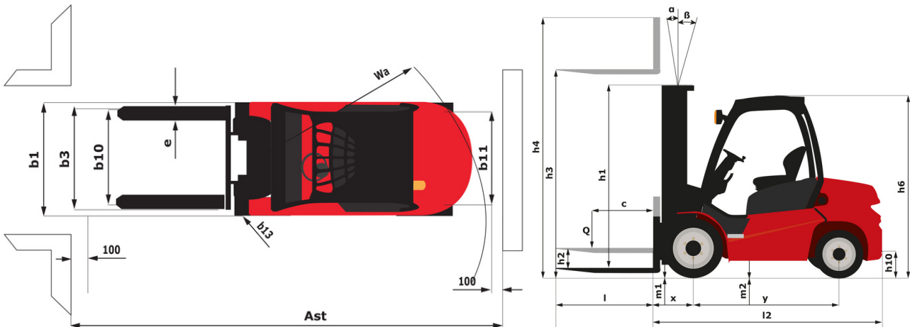
MI 35 D - Tekening met afmetingen
